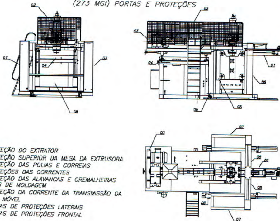
LAY-OUT DIMENCIONAL MAXTEC 30L (273 MGI) PORTAS E PROTEÇÕES
